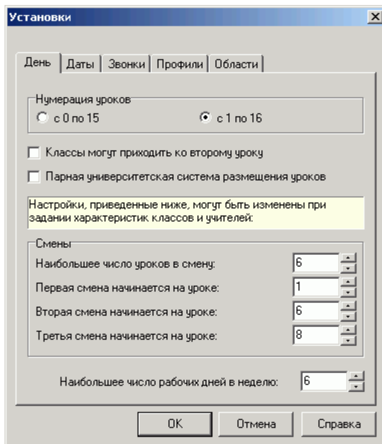
Рисунок 1. Диалог «Установки»
