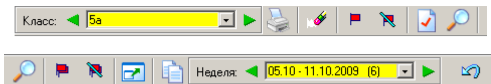
Рисунок 6. Панель инструментов
